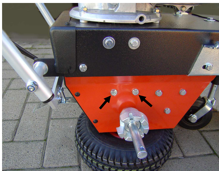
Abbildung 7: Blattfeder-Einstellung
